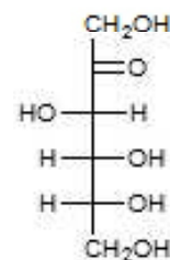
D-Fructose
