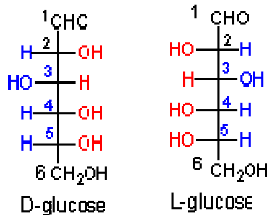
Enantiomers
