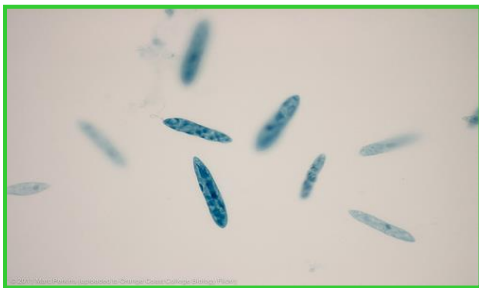
Euglena
