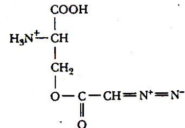
Azaserine O-diazoacetylserine
