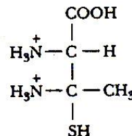
Penicillamine
