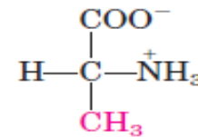
D-Alanine
