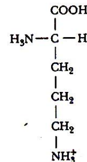
Ornithine
