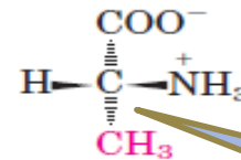
D-Alanine
