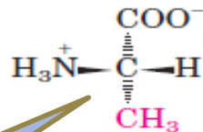
(b) L-Alanine
