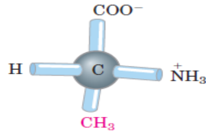
D-Alanine
